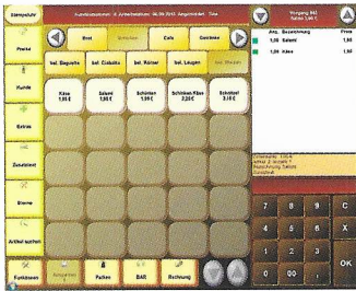
Benutzeroberfläche
