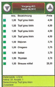
Vorgangsübersicht
